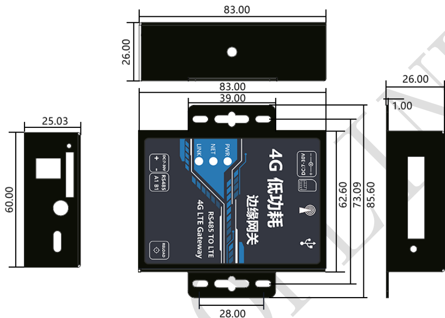
图 3 低功耗 DTU 机械尺寸图 (TOP View)
