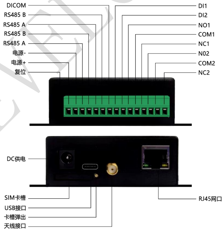
图 1 ZL412ERTU 环保网关插针引脚图（TOP View）
