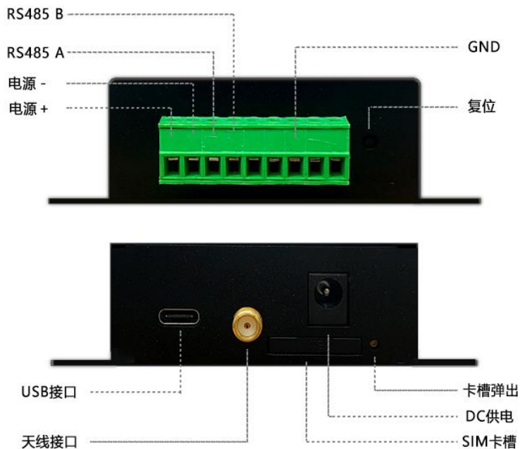
图 1 SL651 水文网关 RTU 插针引脚图 (TOP View)
