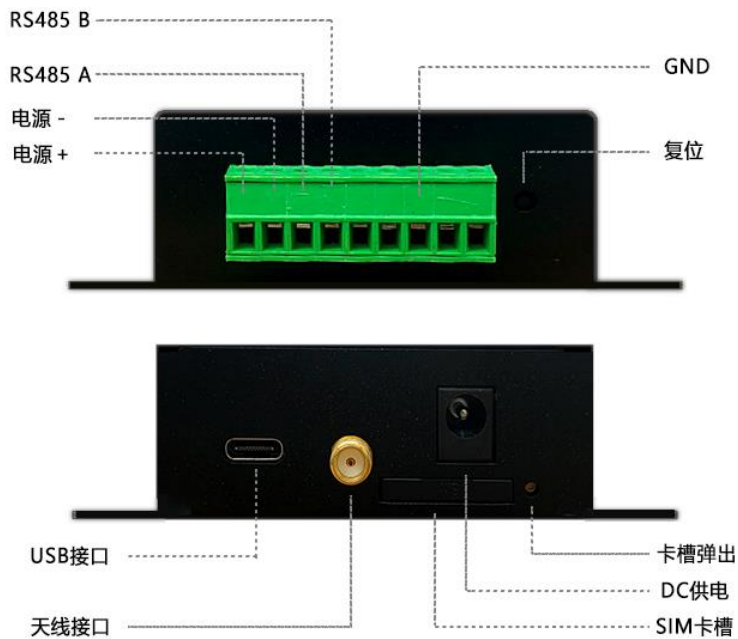
图 1 SZY206 水资源网关 RTU 插针引脚图 (TOP View)
