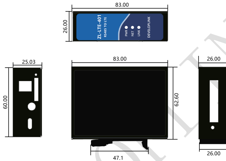
图 2 ZL-LTE-401 导轨 DTU 机械尺寸图 (TOP View)
