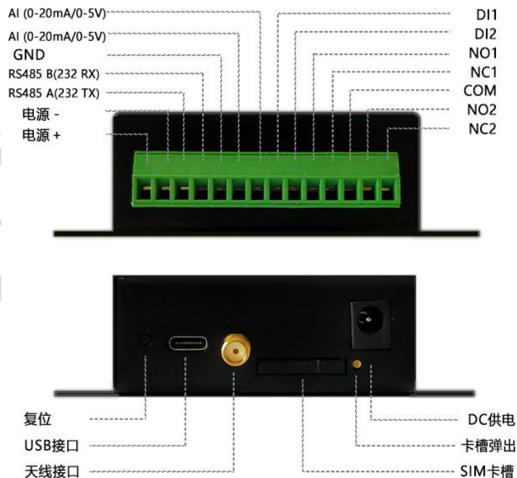
图1 ZL420RTU 插针引脚图 (TOP View)
