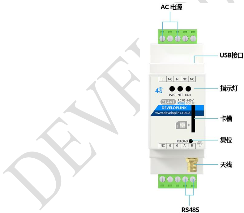
图 1 ZL441 DTU 外部接口图 (TOP View)
