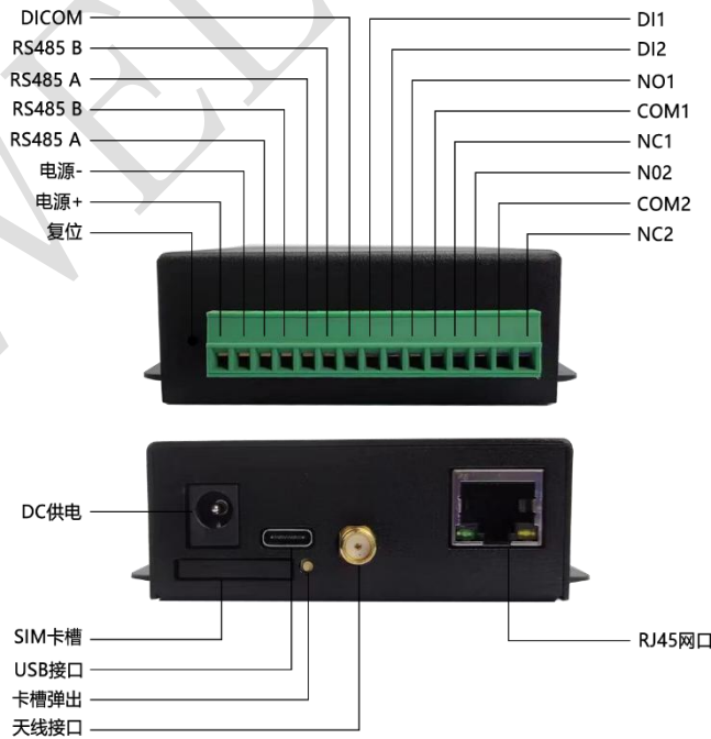
图 1 ZL450RTU 插针引脚图 (TOP View)
