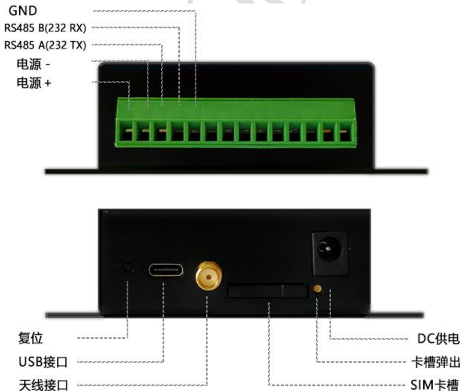
图 1 ZL462 DTU 插针引脚图 (TOP View)
