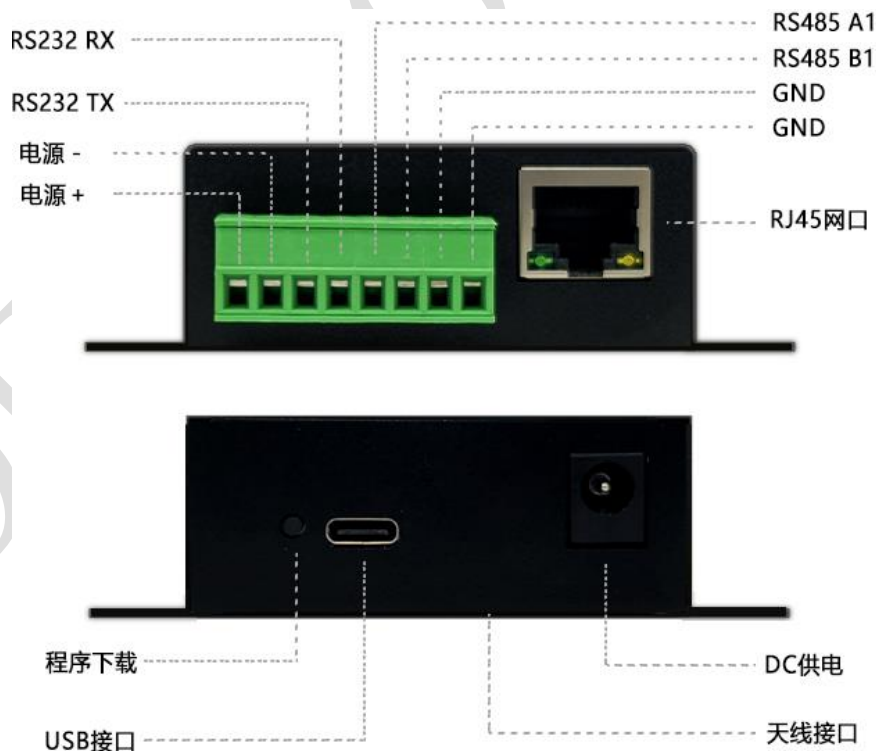
图1 ZL500 DTU插针引脚图 (TOP View)
