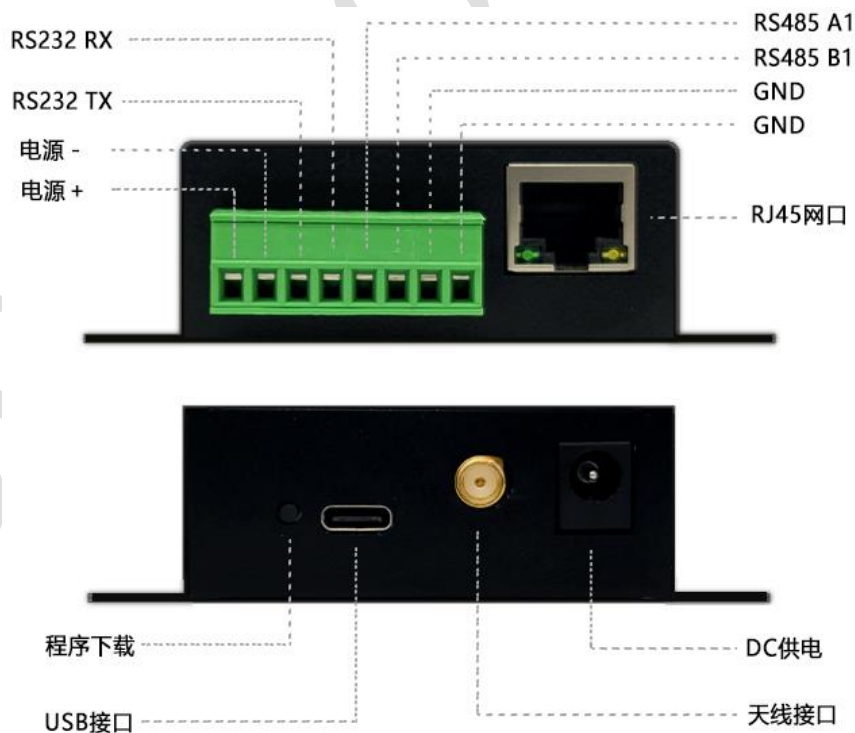
图1 ZL502 DTU插针引脚图 (TOP View)
